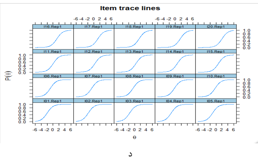
شكل (٢): منحنيات خصائص الفقرة لاختبارات الدراسة عند حجم العينة ١٠٠٠ مفحوص
